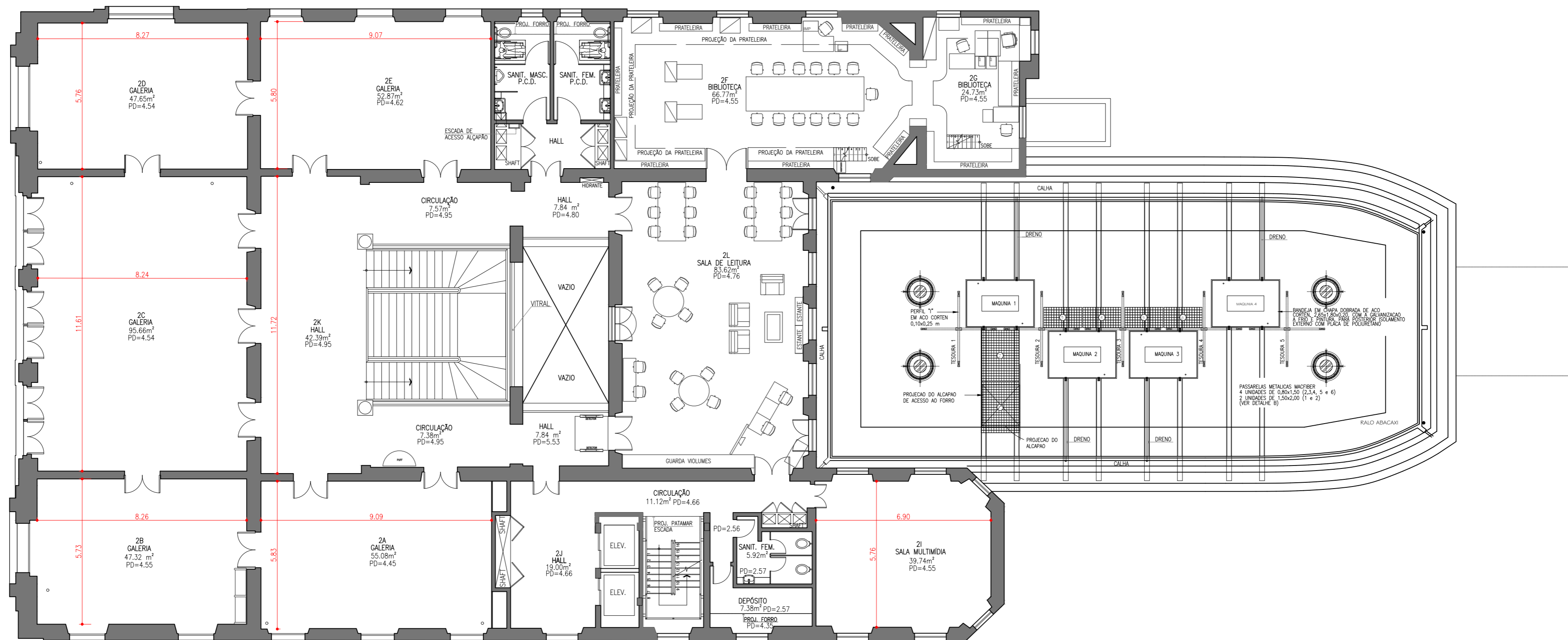
2º PAVIMENTO ESCALA: 1/125
